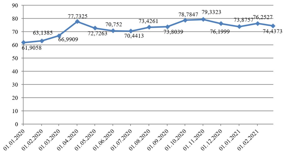
Рис. 7. Динамика курса рубля по отношению к доллару США, руб./долл. США
