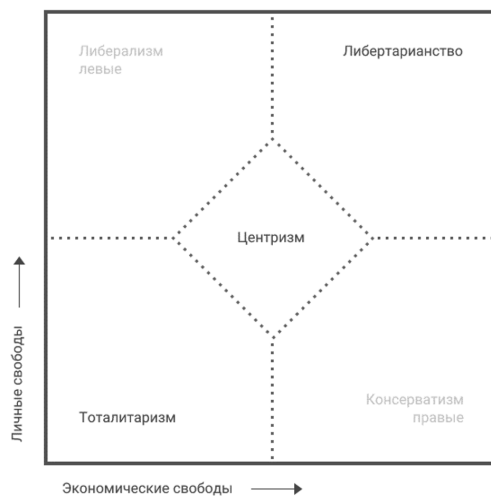
Рис. 1. Диаграмма Нолана
